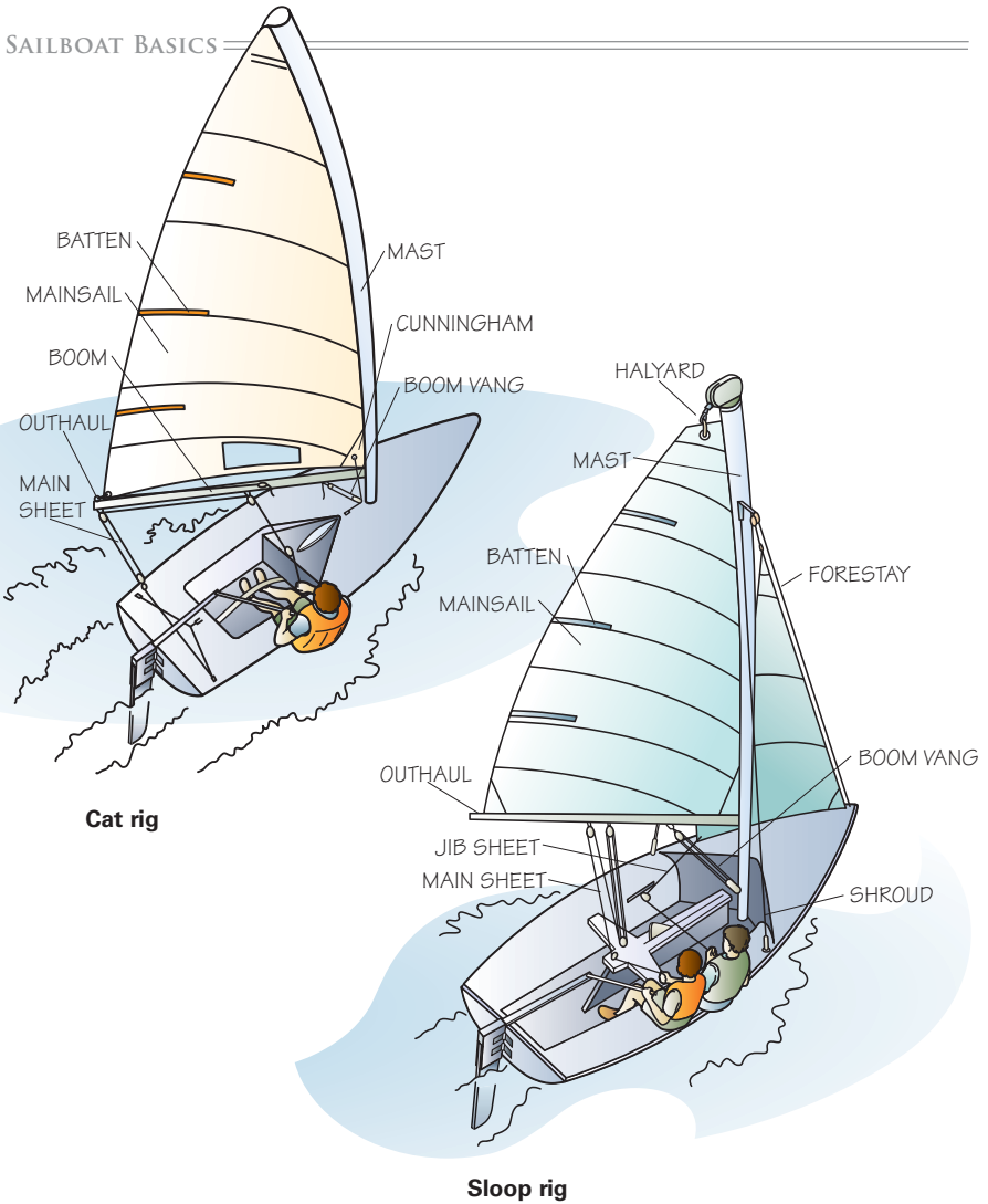
Sloop rig
